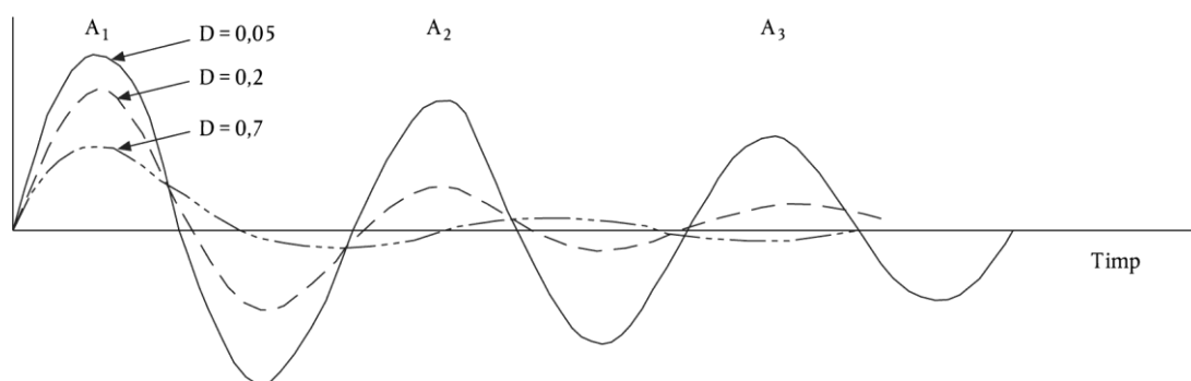
Figura 2 Oscilație tranzitorie amortizată
