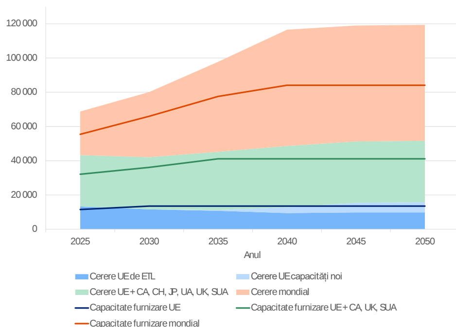
Figura 6 – Cererea globală de servicii de conversie comparativ cu previziunile privind capacitatea de furnizare. (tU ca UF 6 pe an).
