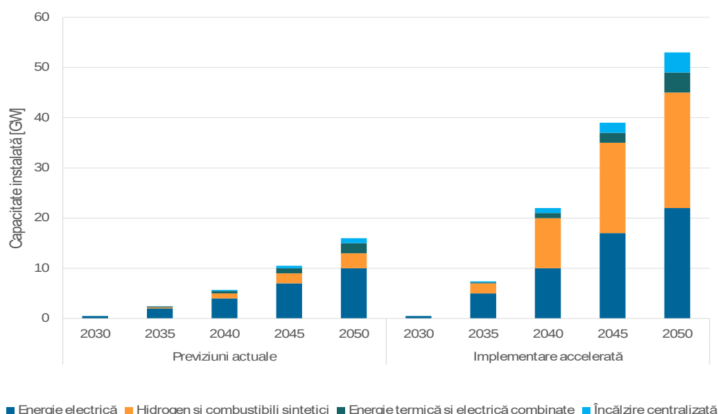
Figura 5 – Scenarii de implementare a SMR cu ponderi ale furnizării de căldură/hidrogen.
