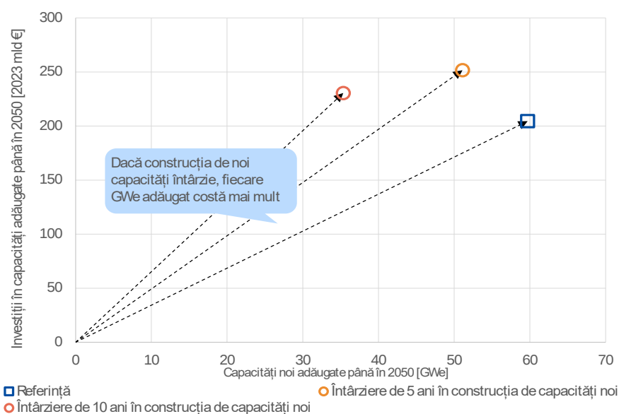
Figura 3 – Nevoile de investiții pentru construcția de noi capacități până în 2050 în cazul scenariilor de întârziere a implementării noilor capacități.
