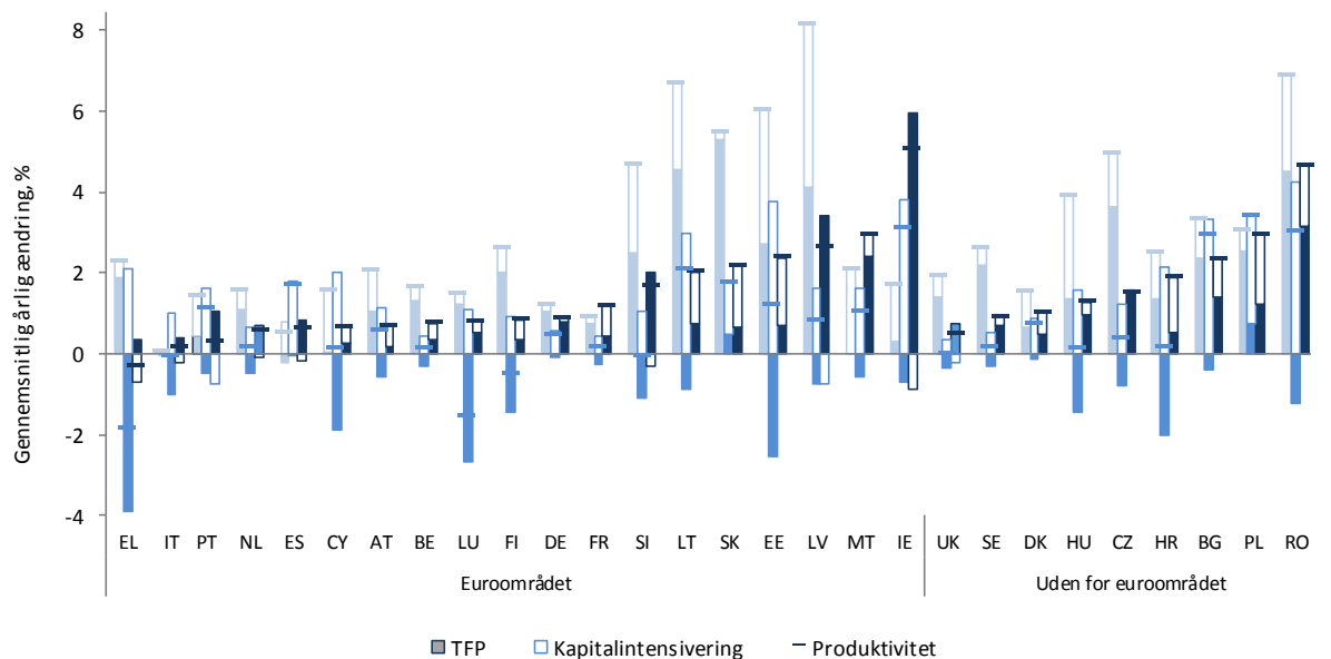
Figur 14: Produktivitetsvækst, delkomponenter, 2002-2018
