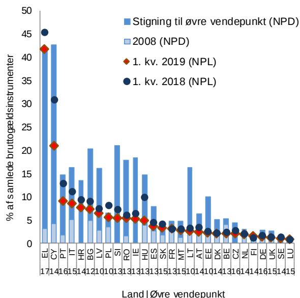
Figur 23: Misligholdte lån
